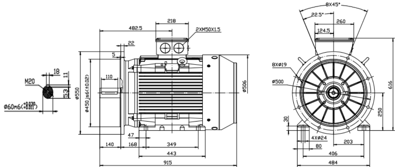
Typ / type IE3 SEV- 250M-2
