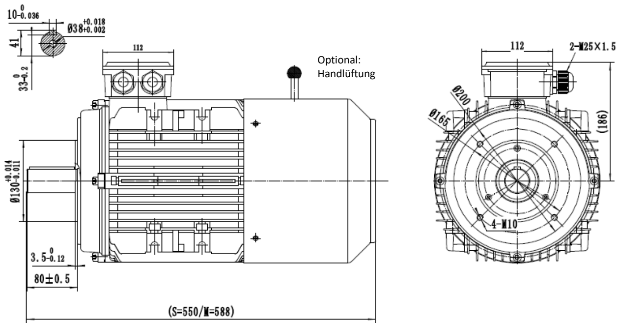
Typ / type SEV-BM3 132S-4
