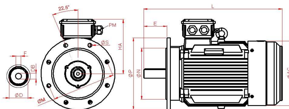
Maßblatt Drehstrommotor / dimensions three phase motor IM B5 [mm]
