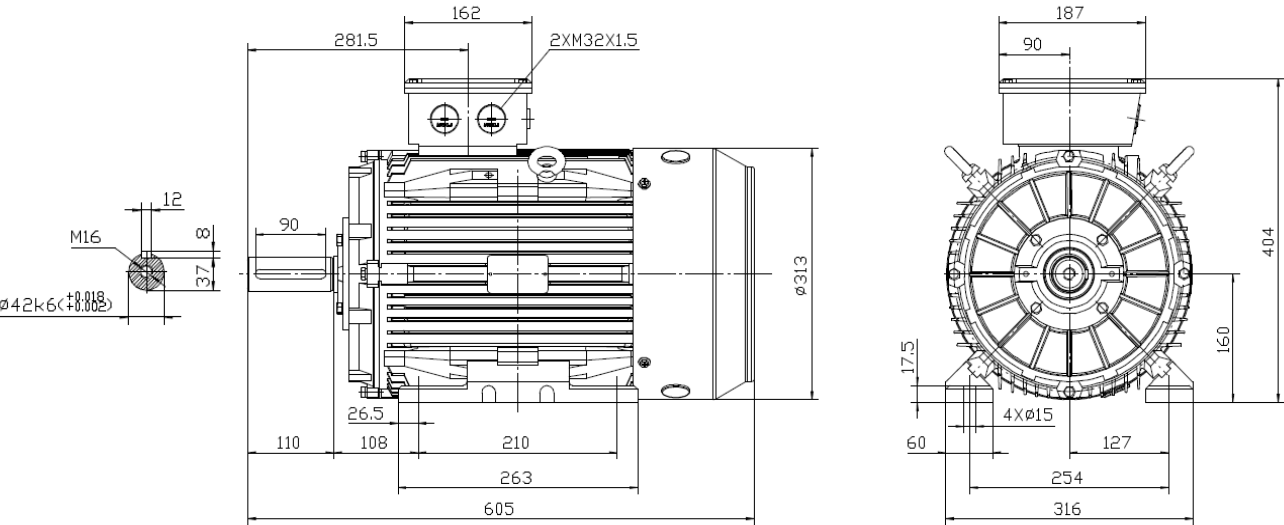
Typ / type IE3 SEV- 160M1-2
