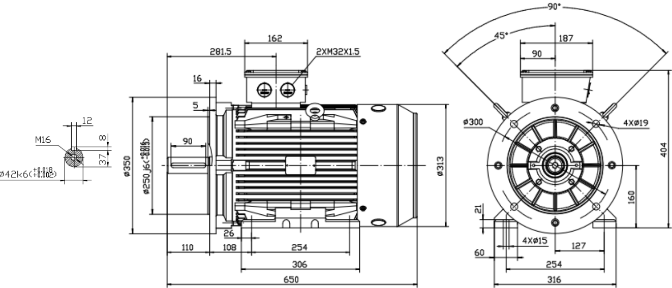
Typ / type IE3 SEV- 160L2-2
